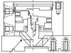
楔形凸轮结构可增加夹持力
