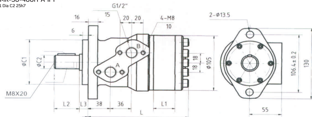
BMR-50-400P*A*II Y BMR-50-400H*A*II Y P1 Dia C2 25h7
