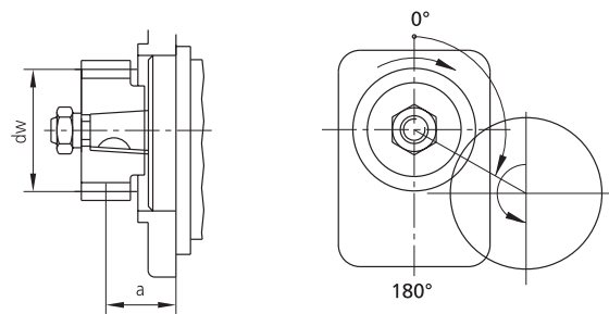
Şekil 3. Dişli ile Tahrık
